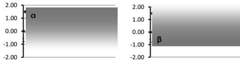
Gambar 10. Visualisasi barisan terbatas di atas dan barisan terbatas di bawah
