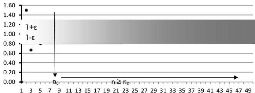
Gambar 4 Visualisasi menentukan dan memberi garis n_0
