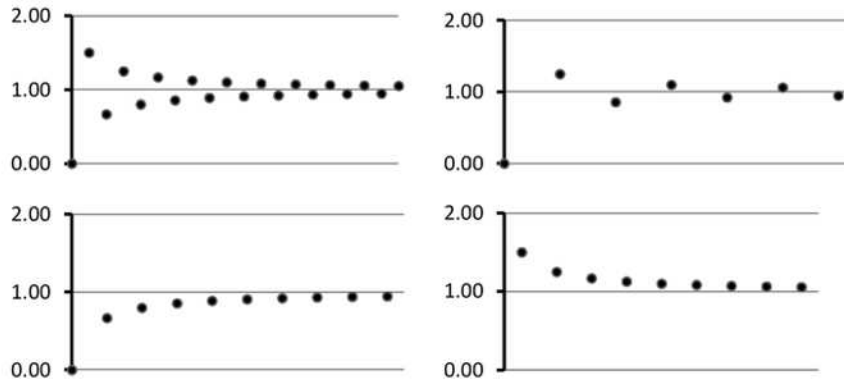
Gambar 11. Visualisasi contoh-contoh subbarisan
