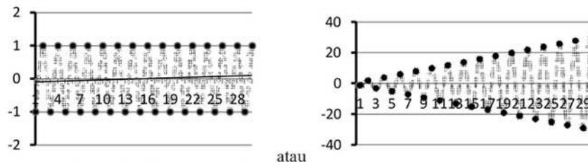
Gambar 6. Visualisasi barisan oscillatori
