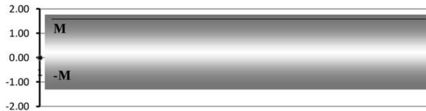
Gambar 9. Visualisasi barisan terbatas
