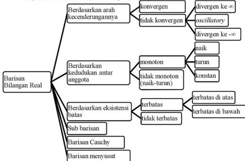
Gambar 1. Hubungan materi barisan bilangan real
