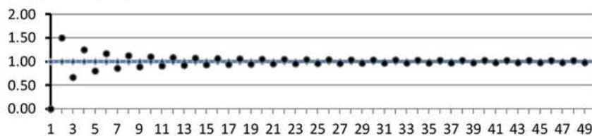
Gambar 2. Visualisasi barisan konvergen
