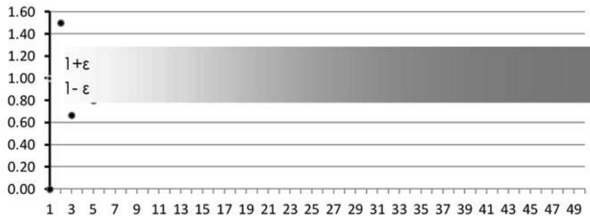
Gambar 3. Visualisasi menentukan dan memberi garis a dan \varepsilon
