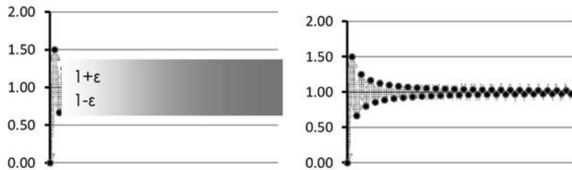
Gambar 12. Visualisasi barisan Cauchy dan barisan menyusut
